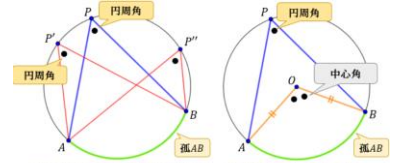
① 同じ弧に対する円周角は等しい ② 円周角=中心角の半分
